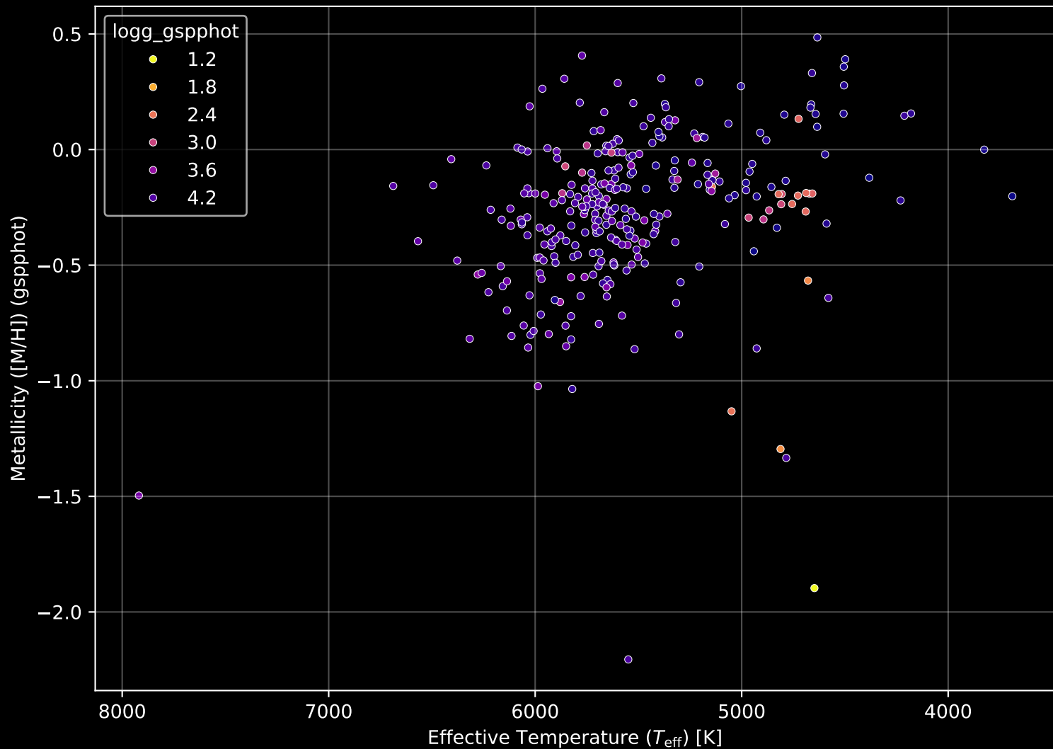
GALAH DR4 Field: [7046] Stellar Population Parameters (n= 298)
